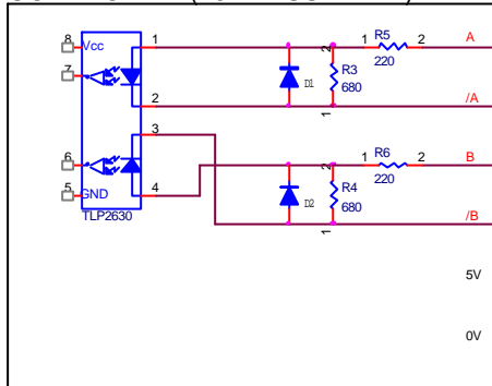
CONTROLLER(25 D-SUB )
